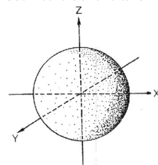
Geometría del Orbital s
