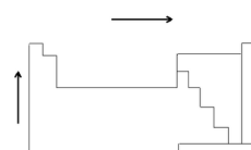
Variación periódica de la electronegatividad.
