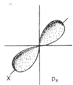
Geometría de un orbital p.
