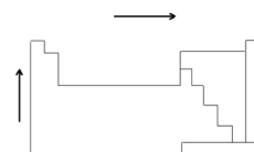
Variación periódica del potencial de ionización.
