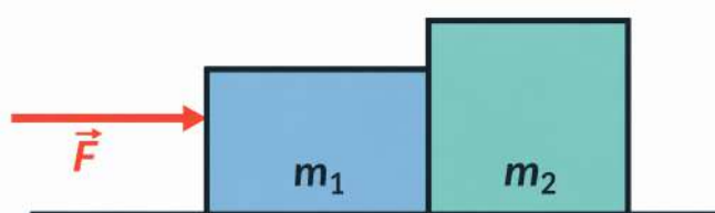
Figura 4.14: Bloques en contacto sobre superficie horizontal para el Problema 1.
