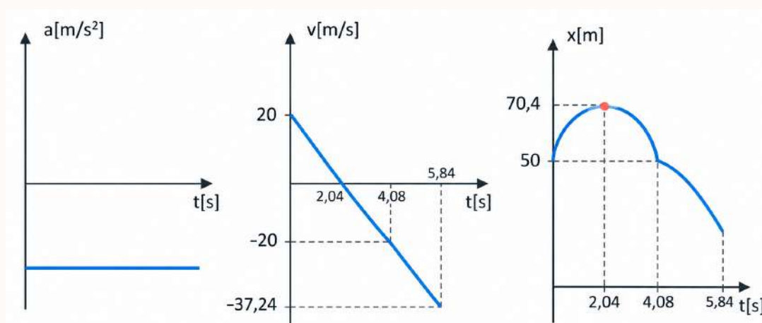
Figura 4.12: Gráficas de aceleración, velocidad y posición en función del tiempo para el Ejemplo 3.
