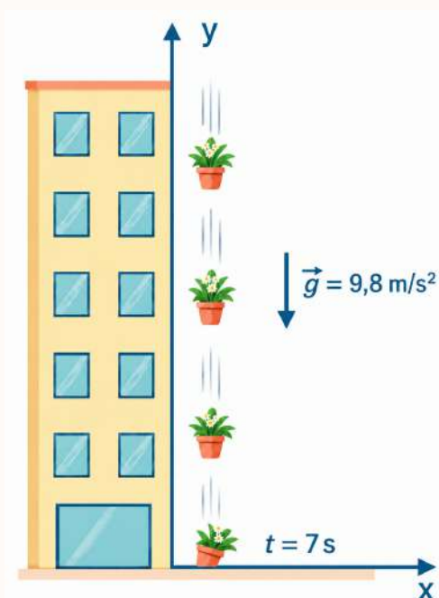
Figura 4.9: Caída libre de una maceta arrojada desde un edificio.
