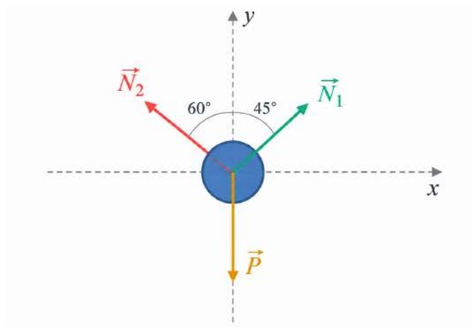
Figura 4.22: Diagrama de cuerpo libre sobre ejes cartesianos para la esfera del Problema 7.
