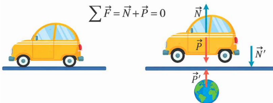
Figura 4.1: Diagrama de fuerzas y pares de interacción en un cuerpo en reposo sobre el suelo.
