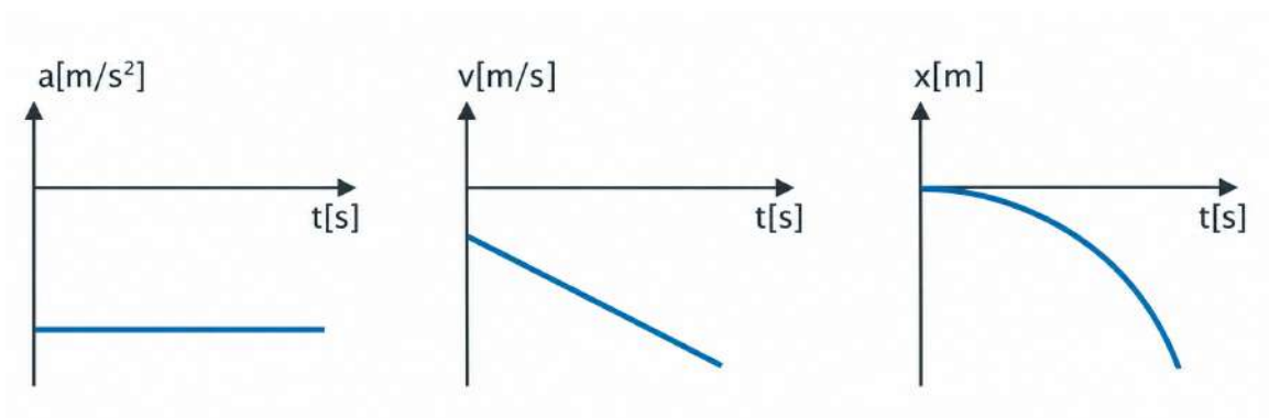
Figura 4.8: Gráficas de aceleración, velocidad y posición en función del tiempo para la caída libre.
