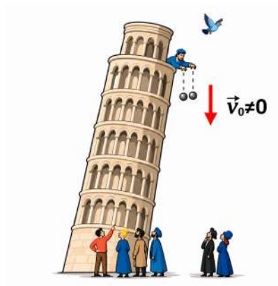
Figura 4.7: Cuerpo lanzado verticalmente hacia abajo con velocidad inicial no nula.
