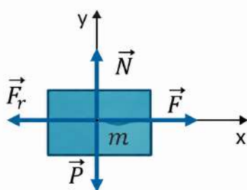
Figura 4.17: Diagrama de cuerpo libre y fuerza aplicada para el Problema 3.
