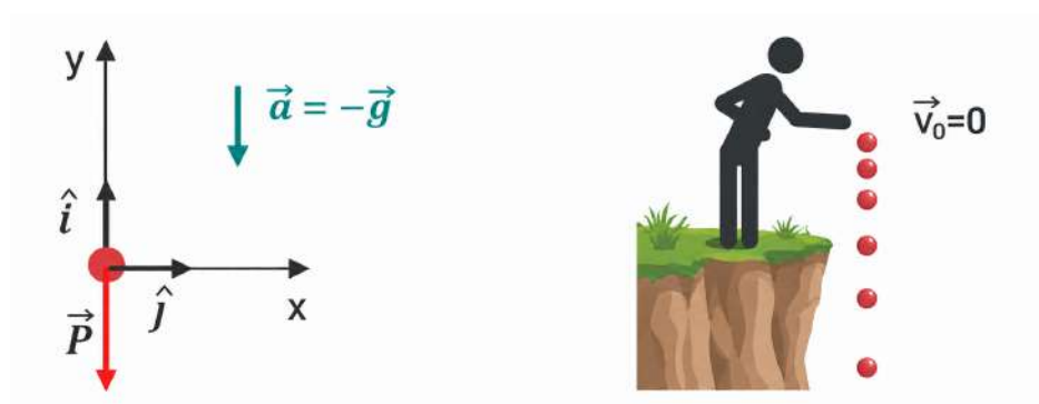
Figura 4.6: Modelo de caída libre en el vacío y diagrama de cuerpo libre.
