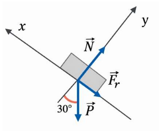
Figura 4.19: Diagrama de cuerpo libre cuando el bloque asciende por el plano inclinado.
