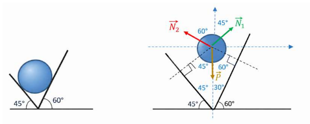
Figura 4.21: Deducción de ángulos y prolongación de fuerzas normales para la esfera entre planos inclinados.
