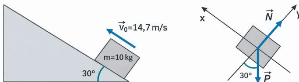
Figura 4.18: Plano inclinado y sistema de ejes rotados para el Problema 5.
