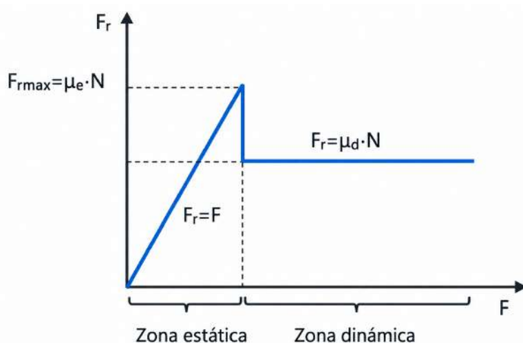
Figura 4.3: Fuerza de rozamiento en función de la fuerza aplicada, distinguiendo las zonas estática y dinámica.
