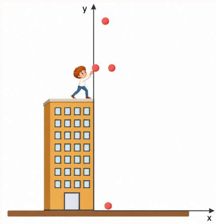
Figura 4.11: Lanzamiento vertical de una piedra desde un edificio de 50 m.
