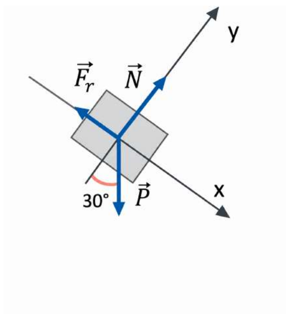
Figura 4.20: Diagrama de cuerpo libre cuando el bloque desciende por el plano inclinado.
