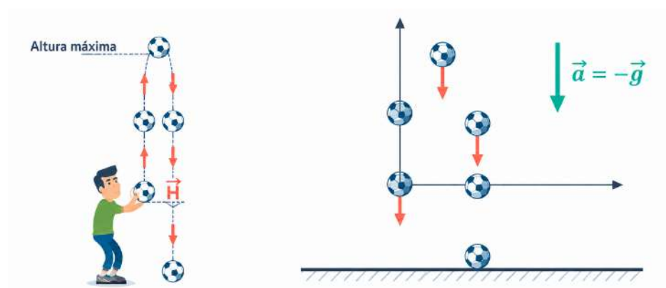
Figura 4.10: Trayectoria y vectores característicos en el tiro vertical.
