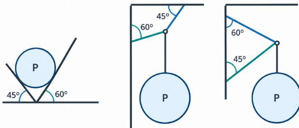
Figura 4.15: Casos de equilibrio estático para el Problema 7.
