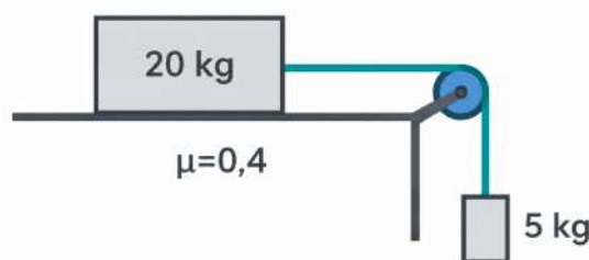
Figura 4.13: Sistema de bloques y polea para la Pregunta 5.
