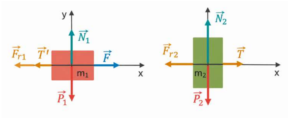
Figura 4.16: Diagramas de cuerpo libre para los cuerpos 1 y 2 del Problema 1.
