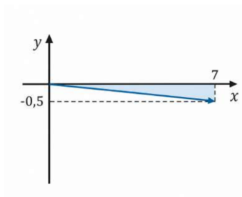
Figura 1.18: Representación gráfica del vector \vec{c} = (7; -0,5) .
