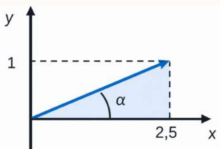
Figura 1.12: Representación gráfica del vector \vec{a} = (2,5; 1) .
