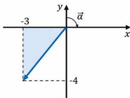
Figura 1.17: Representación gráfica del vector \vec{c} = (-3; -4) .
