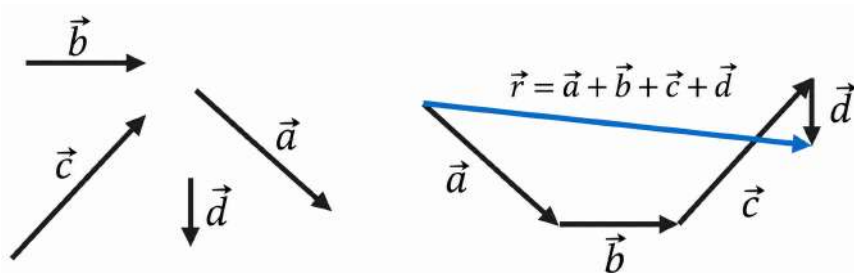
Figura 1.7: Suma geométrica de más de dos vectores: método del polígono.
