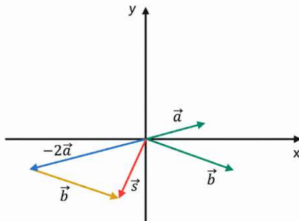
Figura 1.15: Resolución gráfica del vector \vec{s} = -2\vec{a} + \vec{b} .
