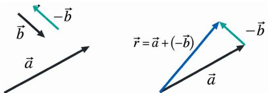
Figura 1.8: Resta geométrica de vectores sumando el vector opuesto.
