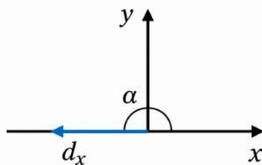
Figura 1.21: Vector \vec{d} sobre el semieje negativo x .
