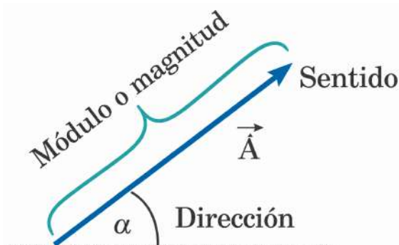
Figura 1.4: Elementos característicos de un vector: módulo, dirección y sentido.
