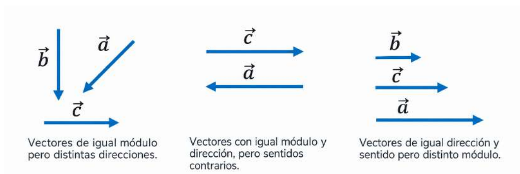
Figura 1.5: Comparación entre vectores: igualdad de módulo, dirección y sentido.
