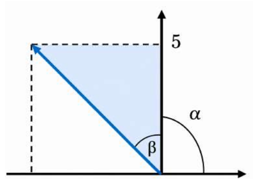
Figura 1.16: Representación gráfica del vector \vec{a} = (-5; 5) .
