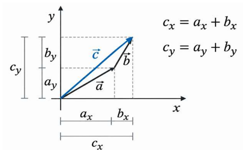
Figura 1.11: Suma analítica de vectores representada en el plano cartesiano.
