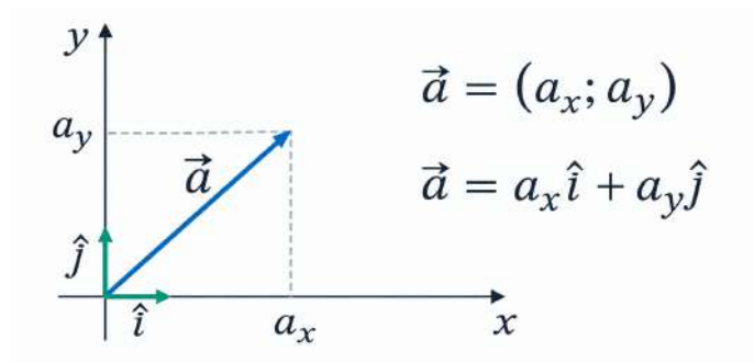
Figura 1.10: Componentes rectangulares y versores canónicos \hat{i} y \hat{j} .
