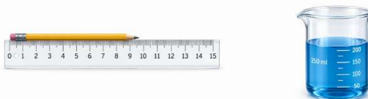
Figura 1.2: Medición de magnitudes escalares: longitud y volumen.
