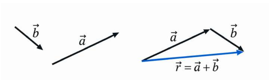
Figura 1.6: Suma geométrica de dos vectores mediante traslación.
